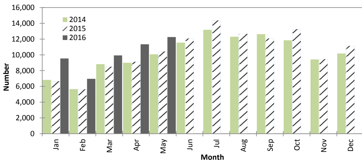
Figure 1: Visitor Arrivals 2014-2016
